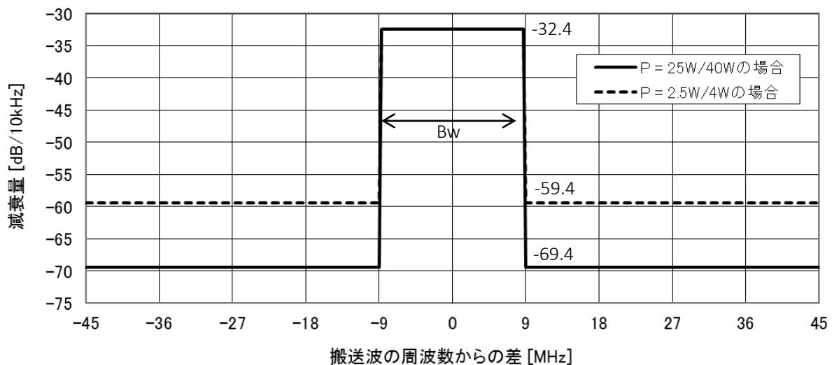
図 4.3.8.3-1 送信スペクトルマスク（フルモード）
