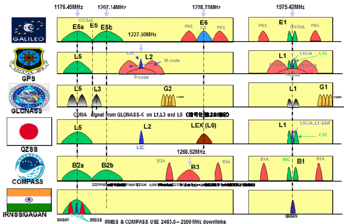
図 4-1 各衛星測位システムの送信信号の周波数分布
