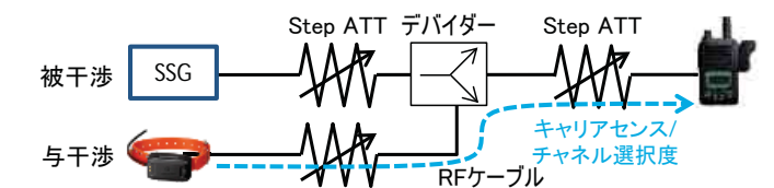
図4-20 測定構成
