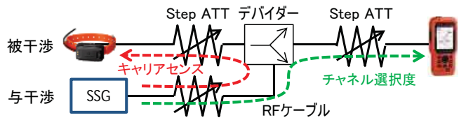
図4-23 測定構成
