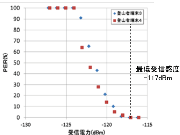
受信電力-PER特性
