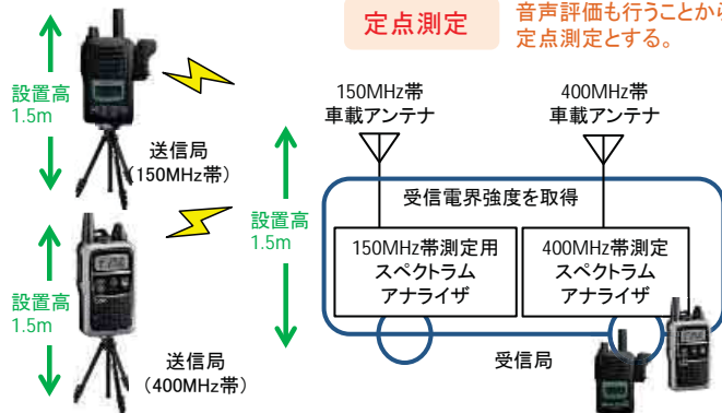
図4-8 測定構成図
