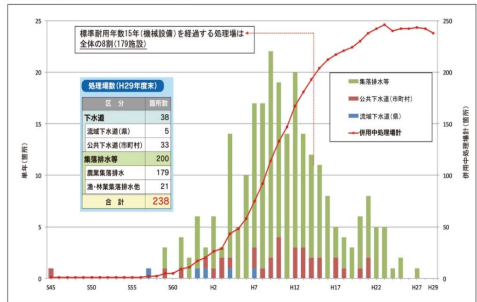
生活排水処理施設 供用処理場数
