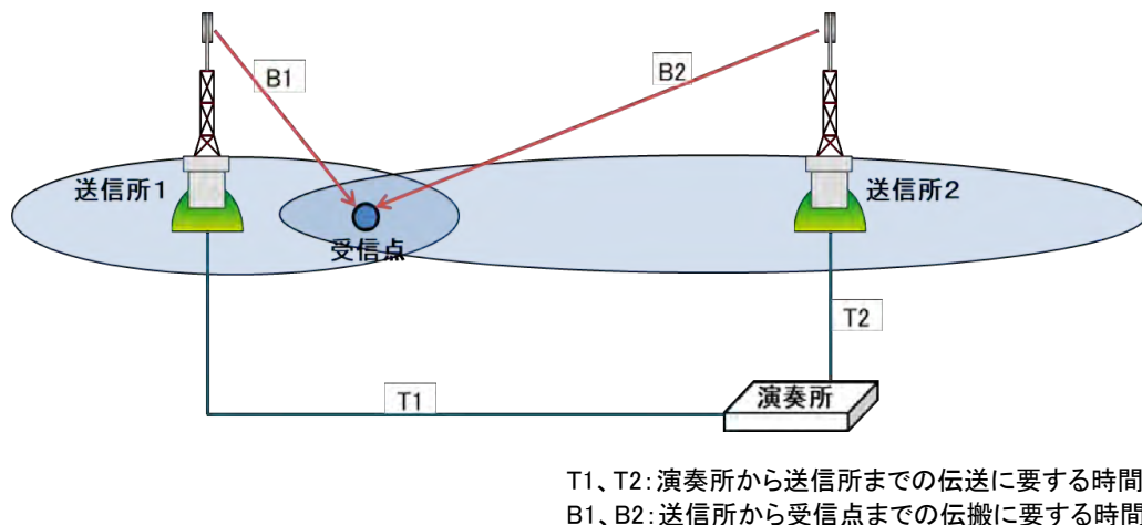
図 3.1.3-1 受信点における遅延時間差の発生
