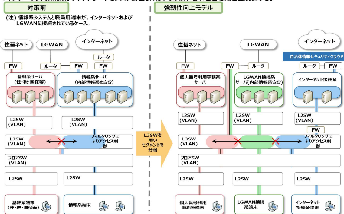
図表 26 強靱性向上モデルにおけるネットワーク再構成の一つのイメージ
